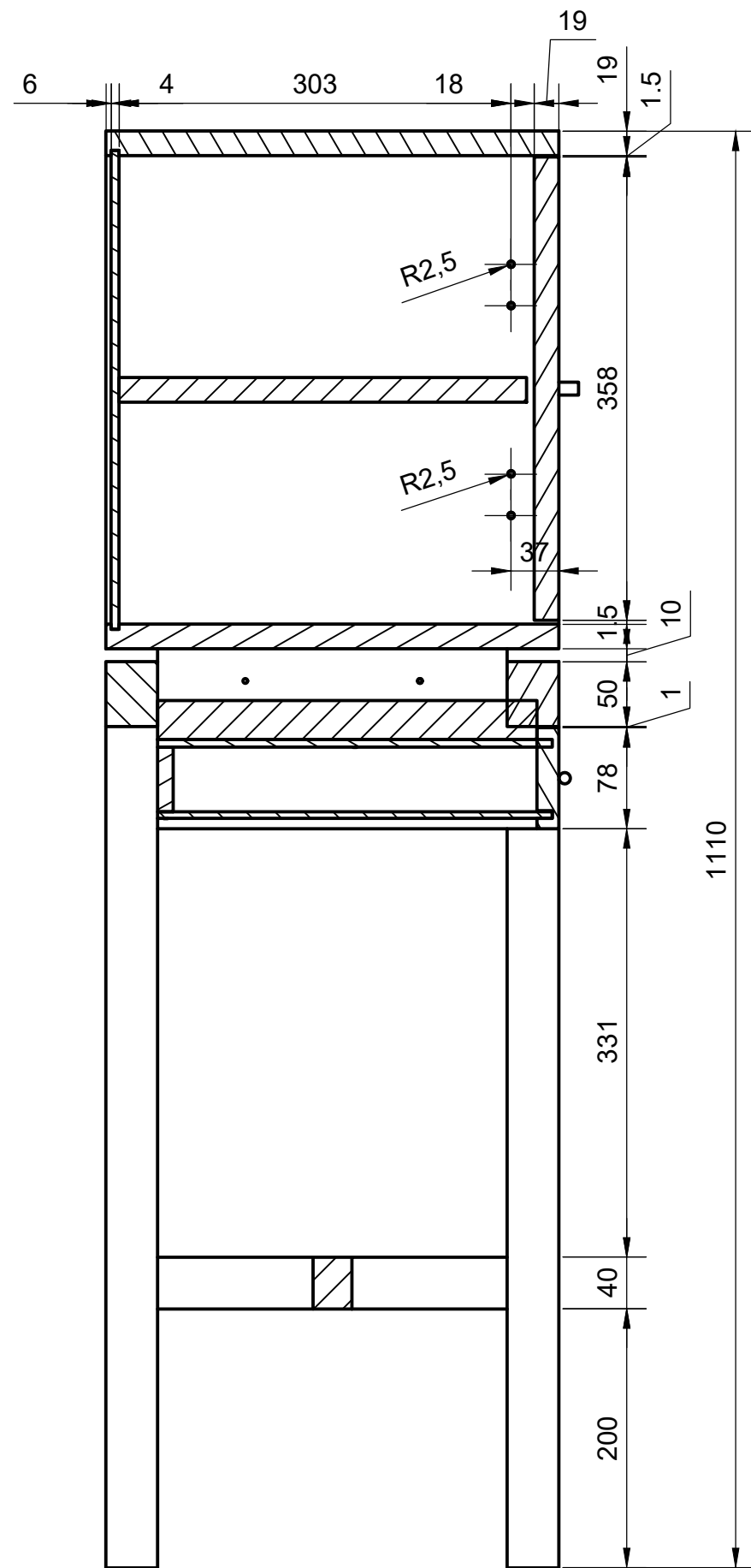
SECCIÓN A-A (1:5)
