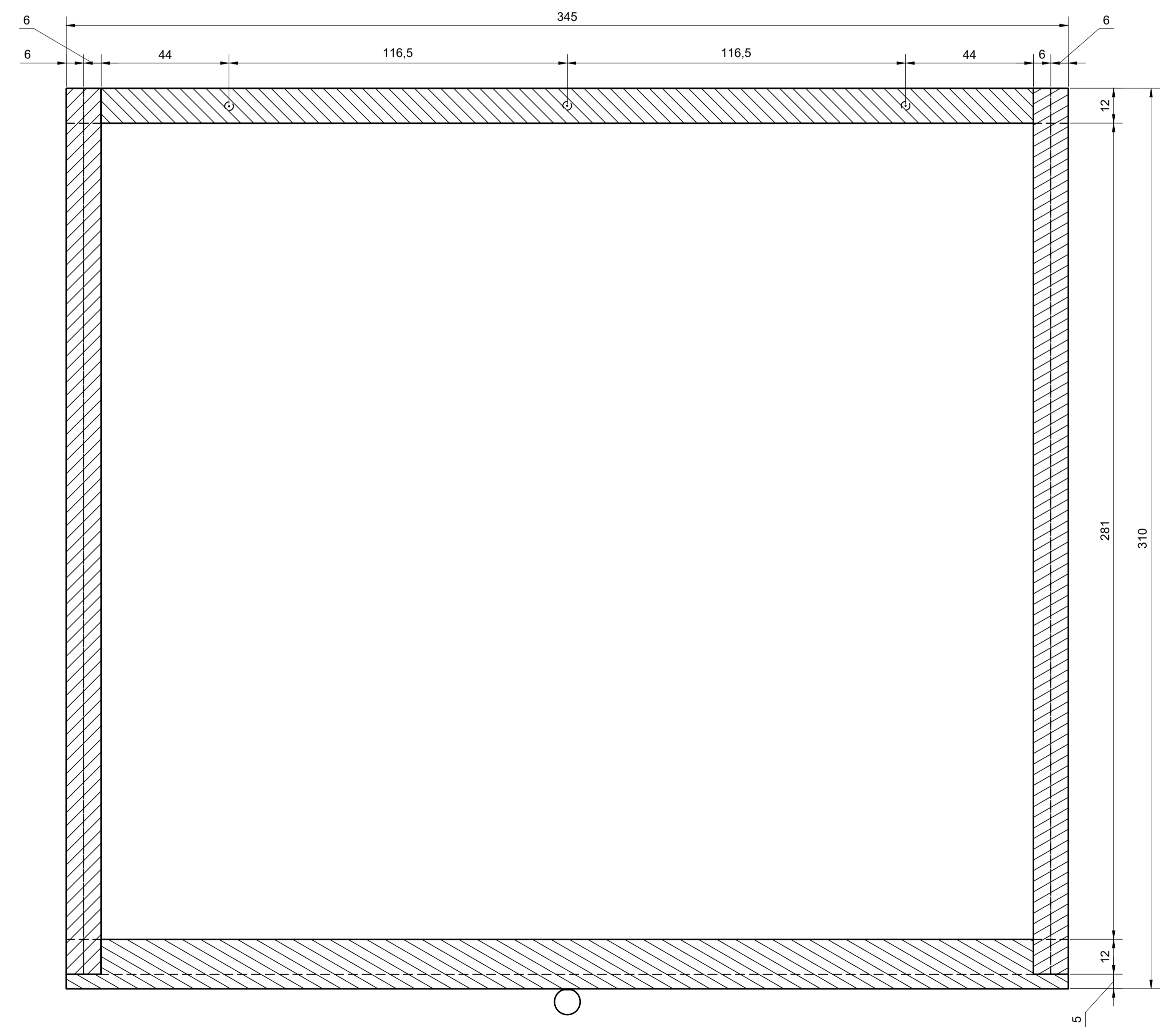
SECCIÓN B-B (1:1)
