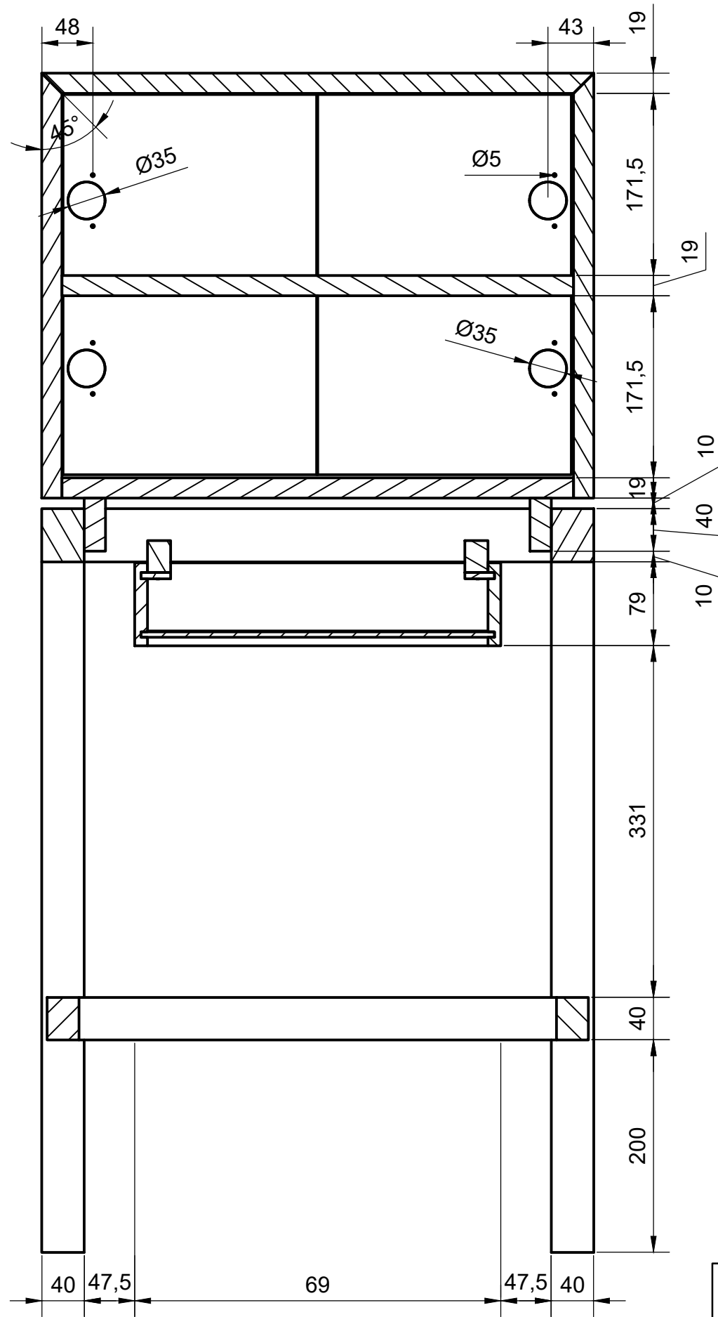
SECCIÓN B-B (1:5)
